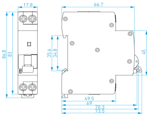
HRO40M, 40 AF
