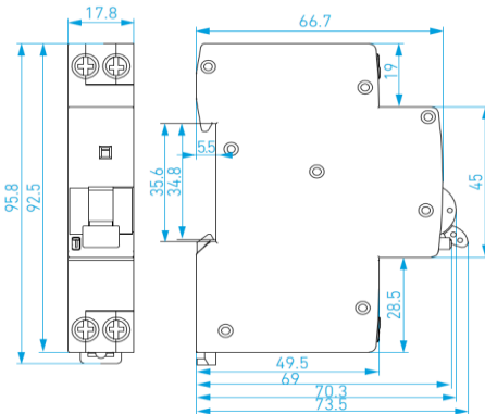
HRO40P, 40 AF
