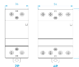
HIC40, 40 AF
