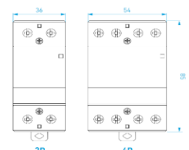
HIC63, 63 AF
