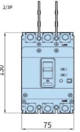
• HGE30, 50E/S, 60, 100
