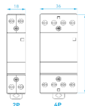
HIC25, 25 AF
